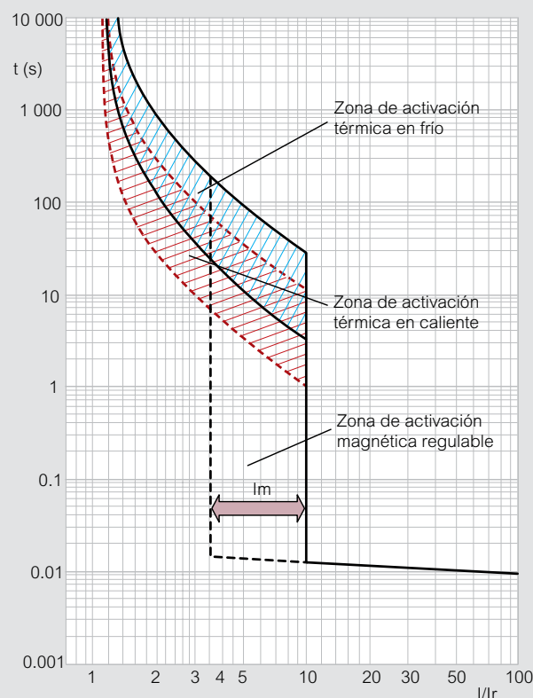
■ Curva de disparo de un DPX 3 termomagnético
