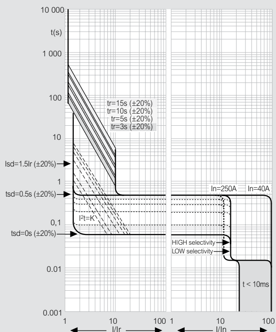
DPX 3 250 electrónico Curvas de disparo
