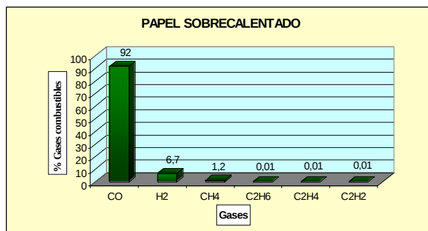
FIGURA 2 PERFIL CROMATOGRAFICO: PAPEL SOBRECALENTADO
