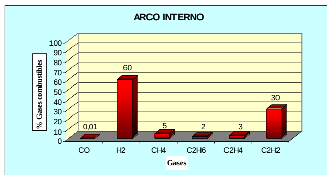
FIGURA 4 PERFIL CROMATOGRAFICO: ARCO INTERNO
