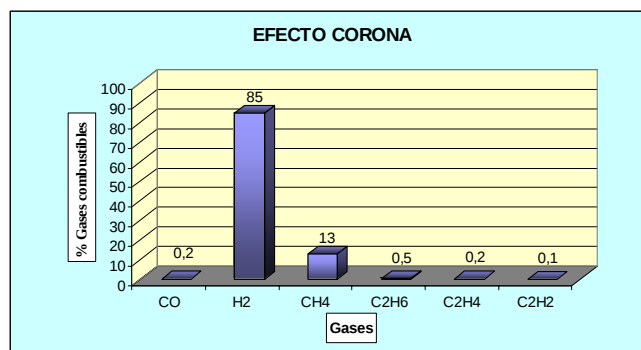
FIGURA 3 PERFIL CROMATOGRAFICO: EFECTO CORONA
