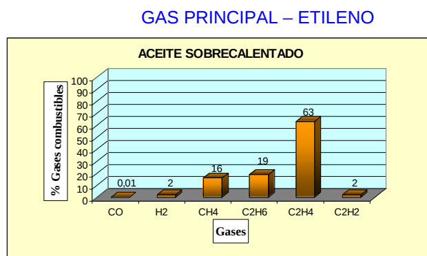
FIGURA 1 PERFIL CROMATOGRAFICO: ACEITE SOBRECALNETADO
